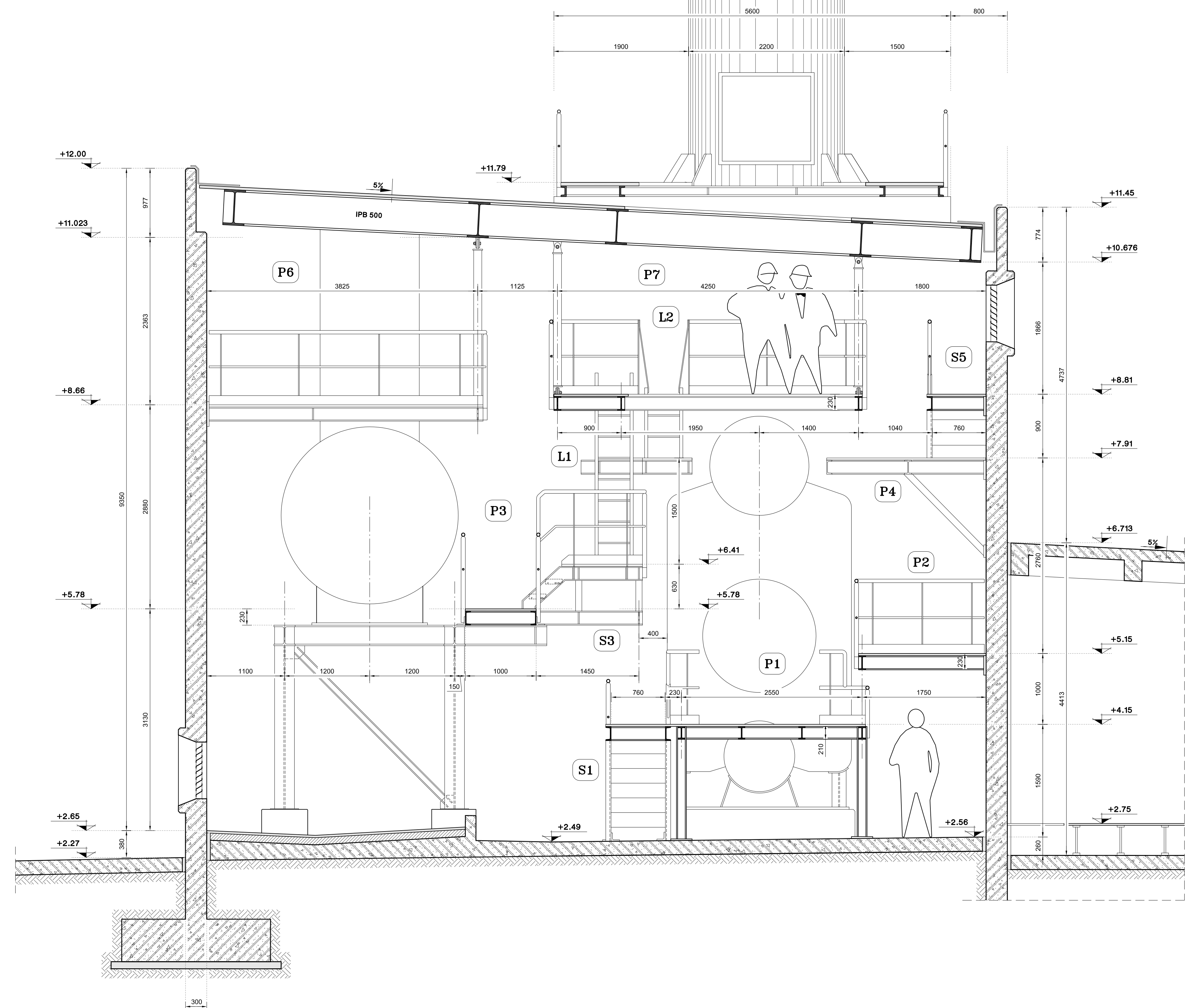
Τομή (2-2)
