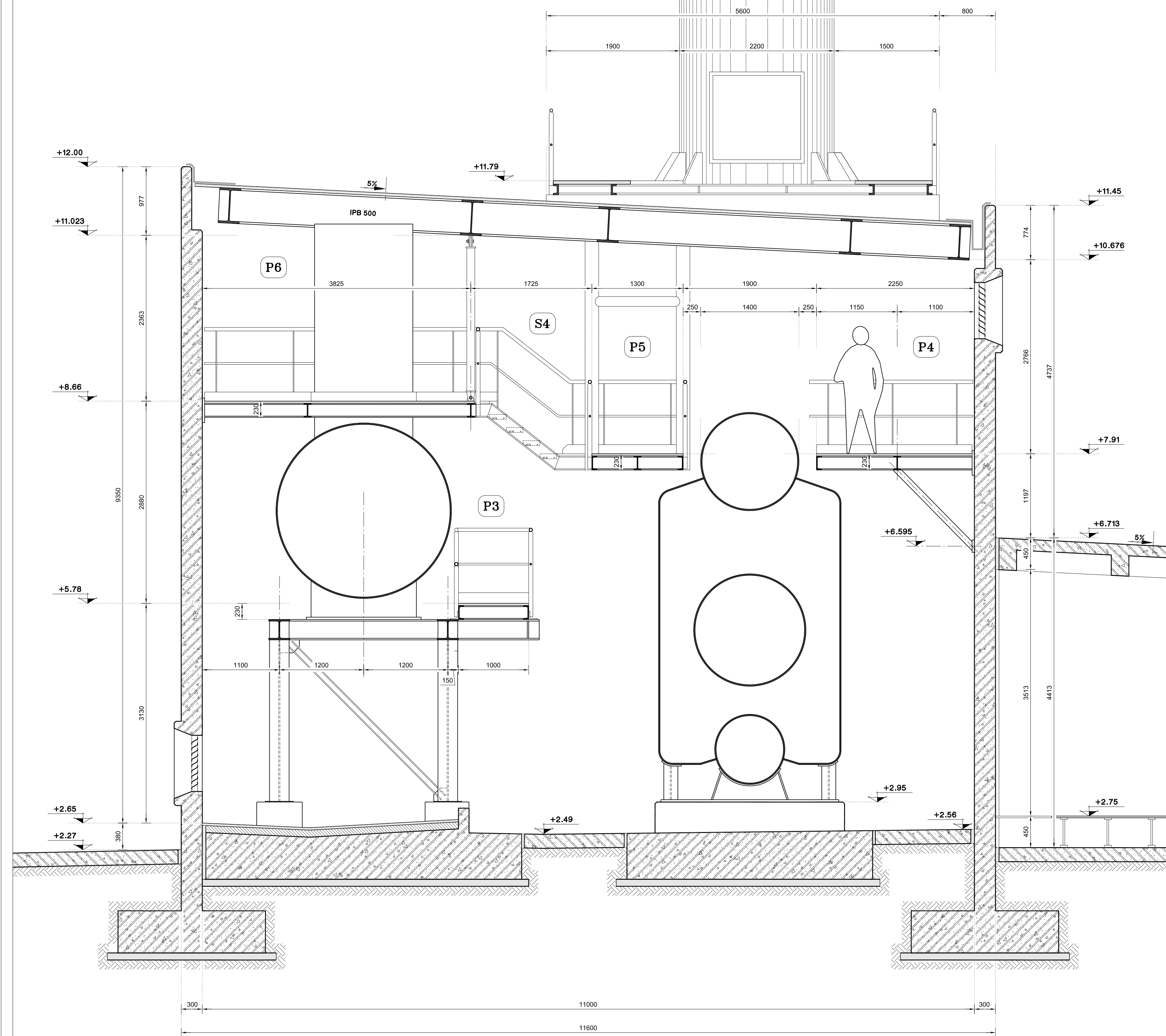
Τομή (1-1)
