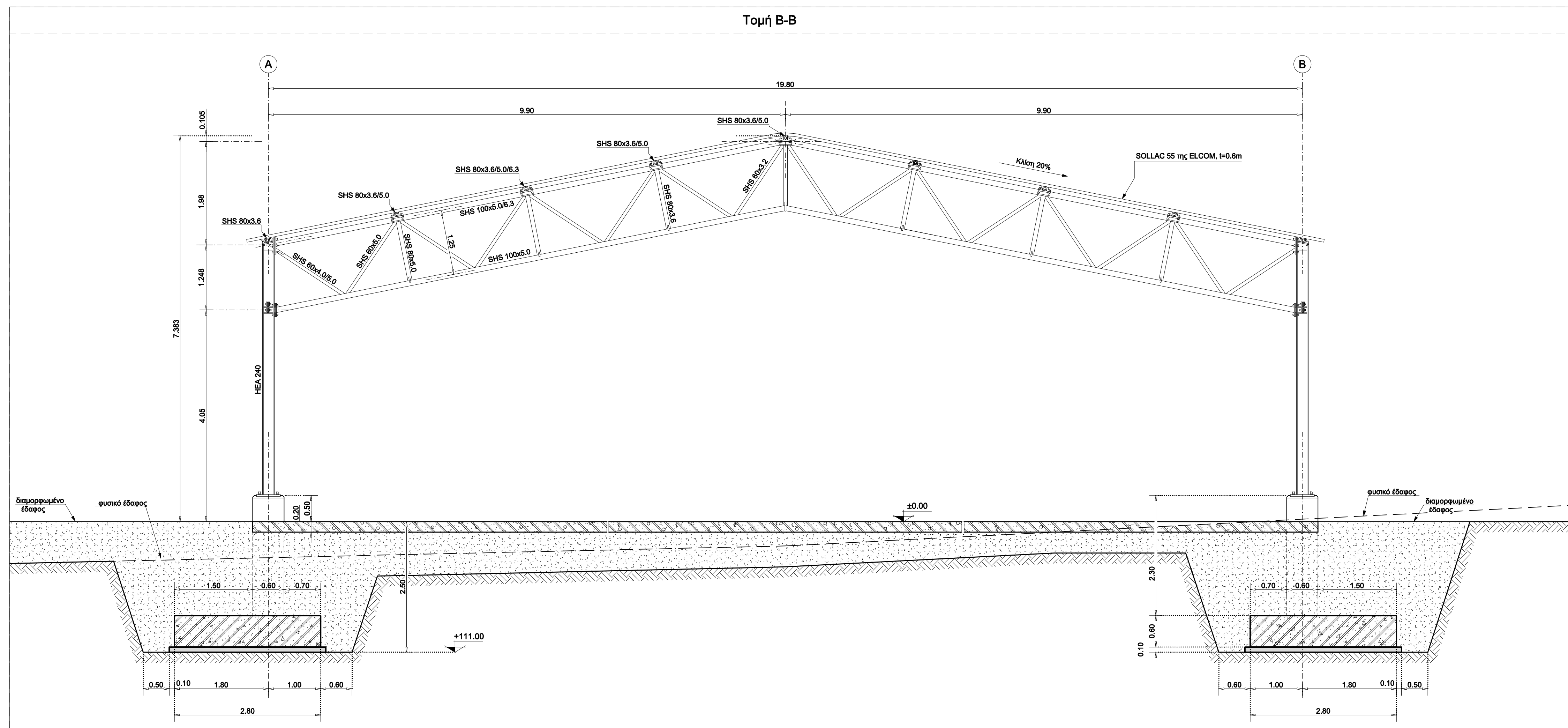
Τομή Γ-Γ
